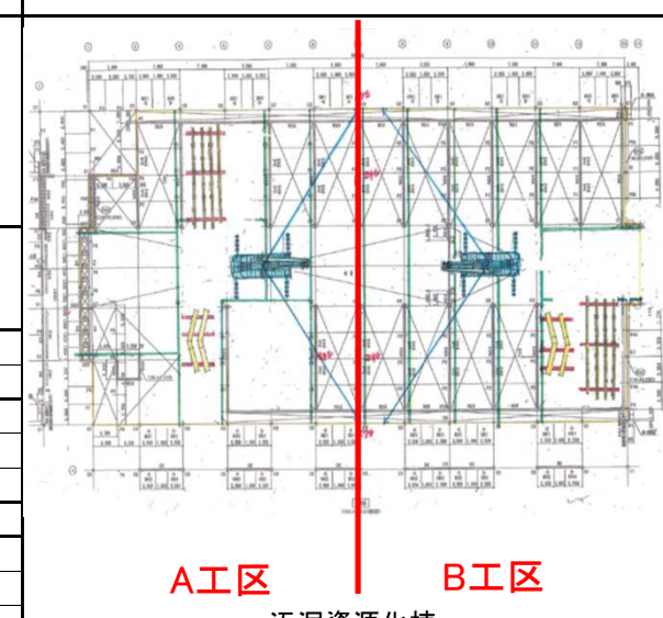
汚泥資源化棟 丸茂・共和・半田 特定JV
